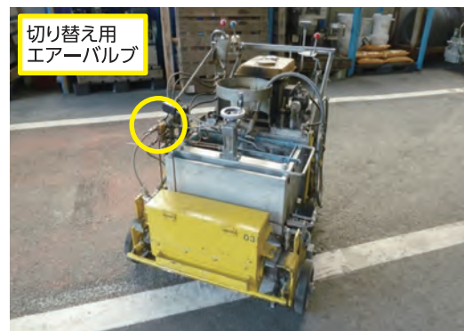
溶融噴射式四輪施工機
