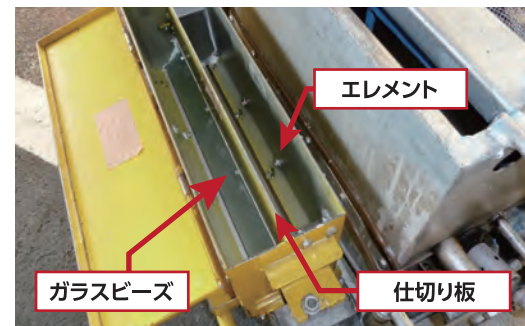
全天候ミストライン用ダブル散布機
