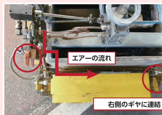
全天候型ミストライン施工時のバルブの向き
