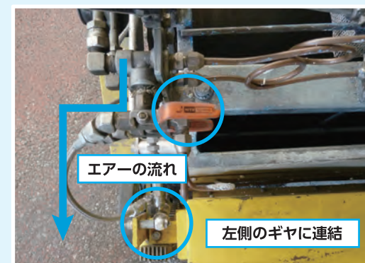
カラーAWT施工時のバルブの向き
