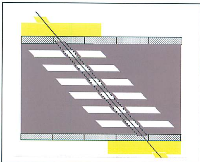
図-1 (○) 正しい設置例
